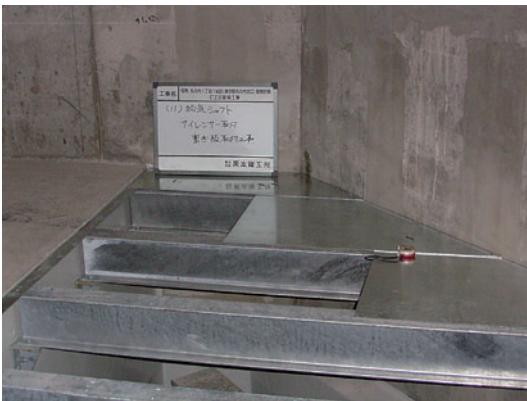
図12 遮音板の施工
