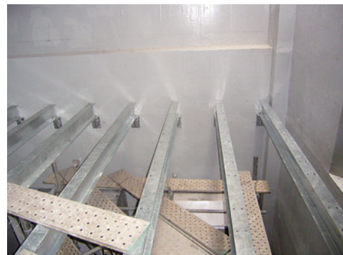
図10 架台取付け
