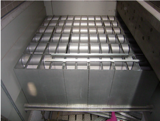
図11 サイレンサ設置
