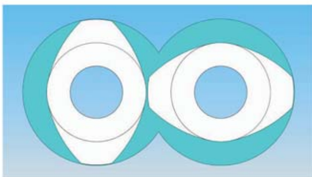
KEXN(当社標準押出機)パドル断面図
