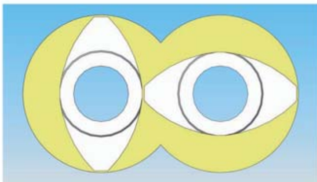
KEXD パドル断面図
